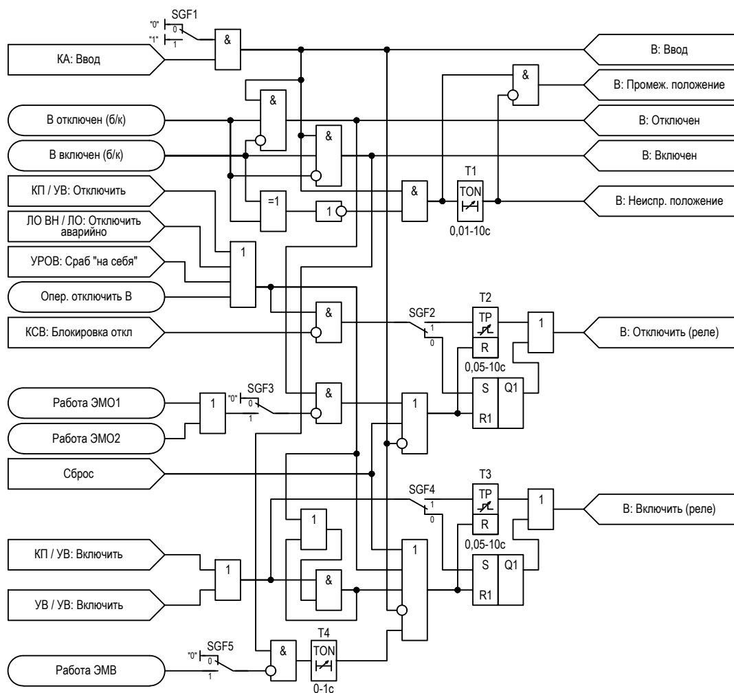
Рисунок 2.27 – Функциональная схема логики выключателя
